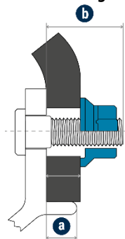
Einzelmontage
