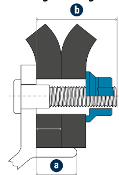
Zwillingsmontage
